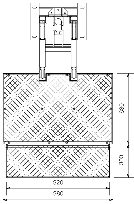
Boven aanzicht
