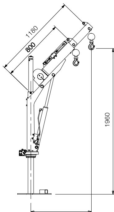
Zij aanzicht
