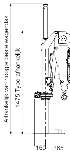
Zij aanzicht ingeklapt
