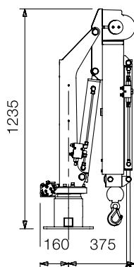
Zij aanzicht ingeklapt
