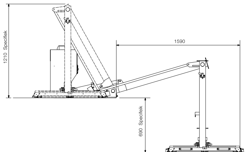
Zij aanzicht
