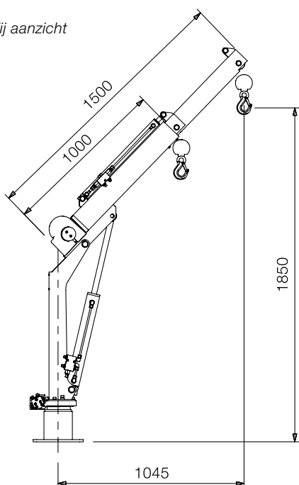
Zij aanzicht
