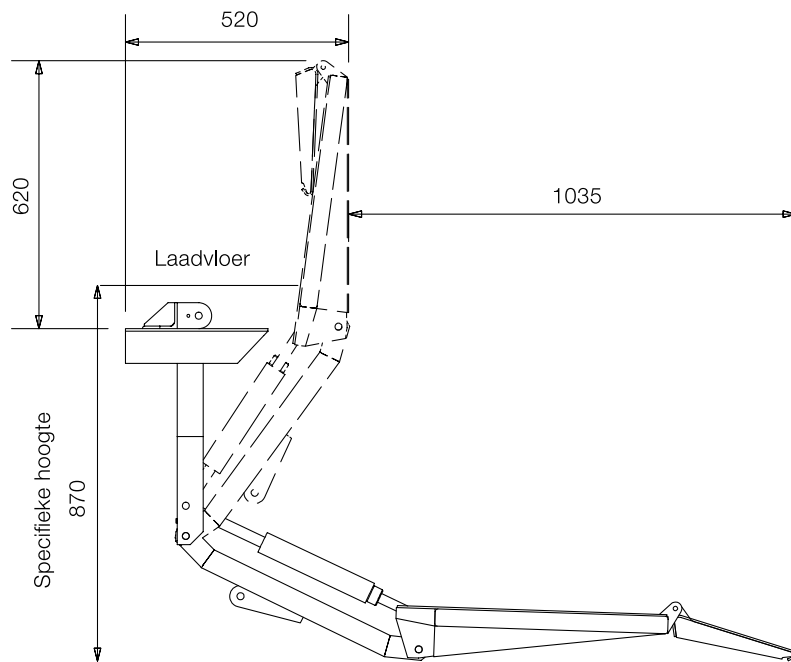
Zij aanzicht
