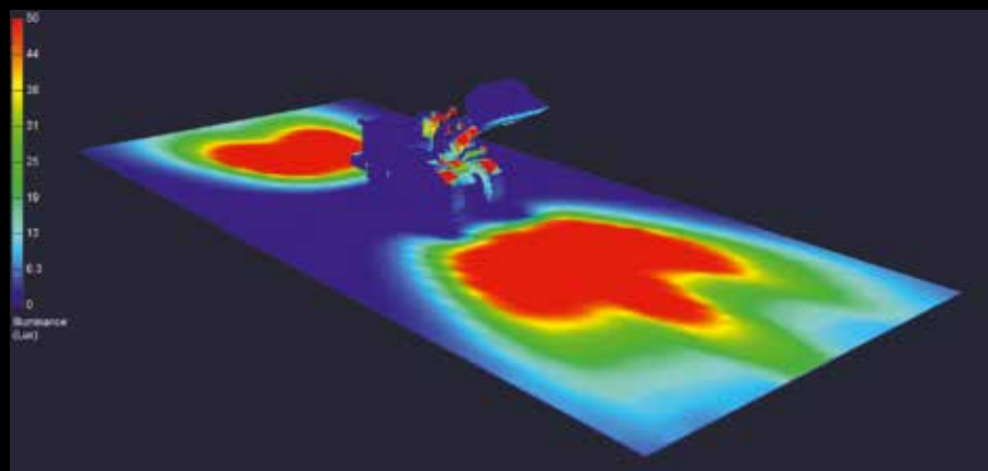
3D Luninantiebeeld
