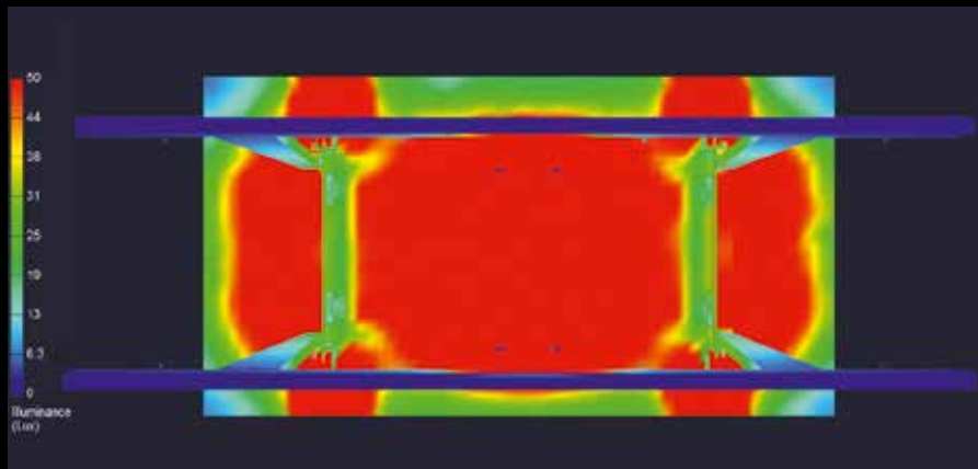
Luninantiebeeld
